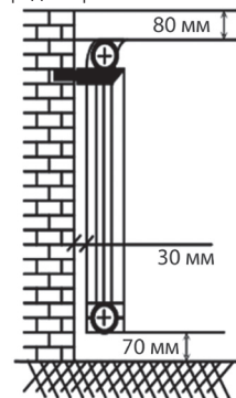
Рис. 2. Правила установки радиатора
