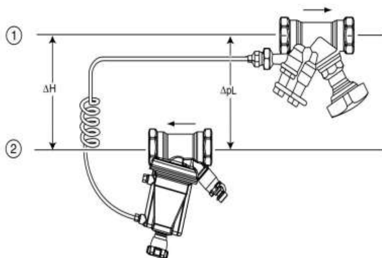
Схема установки
