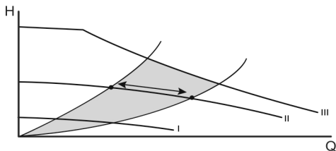
Рис. 14 Пример трёх кривых фиксированных скоростей
