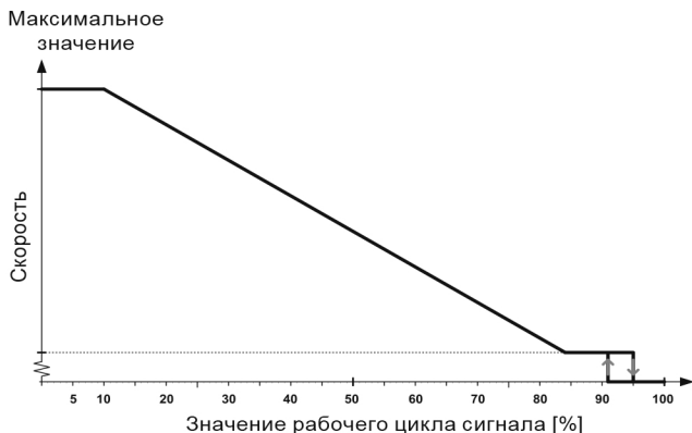
Рис. 16 Профиль «А» входного ШИМ-сигнала в ALPHA1 L
