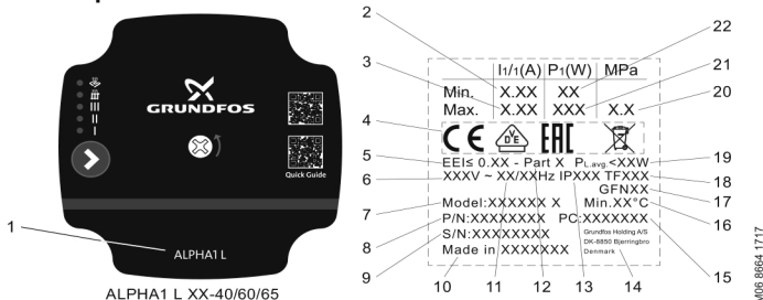
Рис. 1 Фирменная табличка насоса ALPHA1 L
