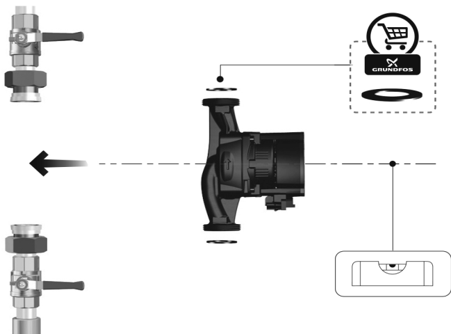
Рис. 3 Монтаж насоса ALPHA1 L
