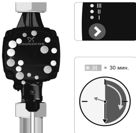
Рис. 10 Удаление воздуха из насоса ALPHA1 L
