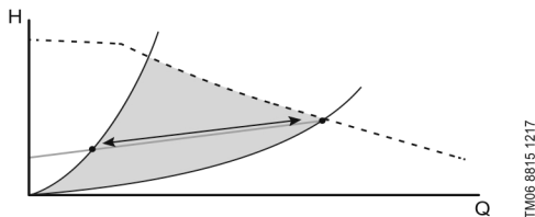
Рис. 12 Пример кривой пропорционального давления в режиме поддержания пропорционального давления
