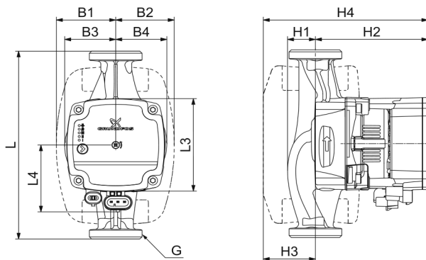
Рис. 22 Габаритные размеры ALPHA1 L XX-60
