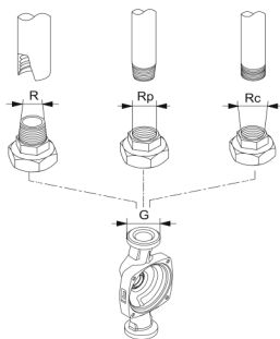
Рис. 26 Резьба G и резьба R
