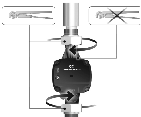
Рис. 4 Затяжка фитингов
