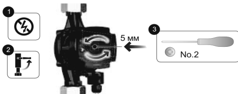
Рис. 25 Разблокировка вала
