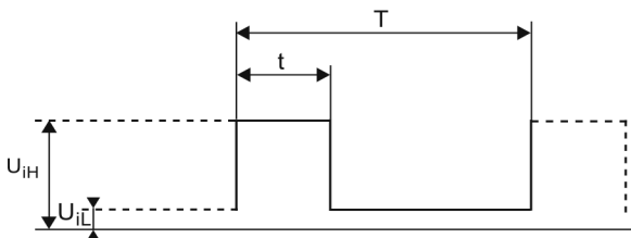
Рис. 15 Иллюстрация ШИМ сигнала
