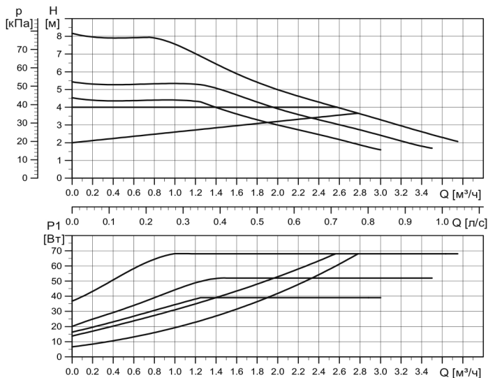
Рис. 23 Расходно-напорная характеристика ALPHA1 L XX-80
