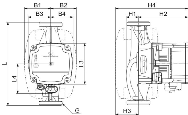
Рис. 20 Габаритные размеры ALPHA1 L XX-40
