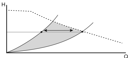
Рис. 13 Пример кривой постоянного давления в режиме поддержания постоянного давления
