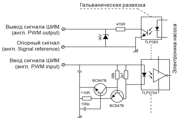
Рис. 18 Электрическая схема интерфейса насоса
