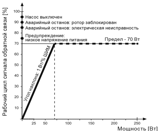
Рис. 17 Профиль ШИМ-сигнала обратной связи
