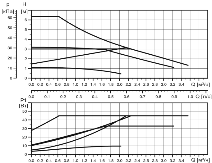
Рис. 21 Расходно-напорная характеристика ALPHA1 L XX-60
