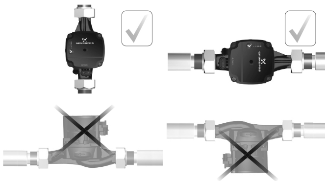
Рис. 5 Расположение насоса ALPHA1 L
