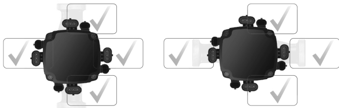
Рис. 6 Расположение головной части насоса ALPHA1 L
