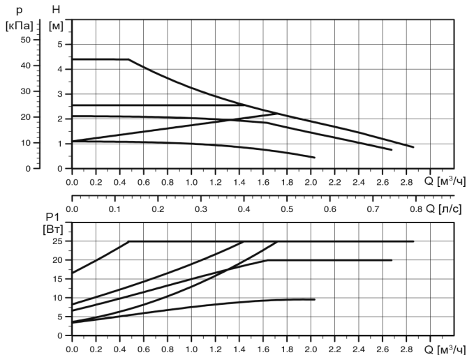
Рис. 19 Расходно-напорная характеристика ALPHA1 L XX-40
