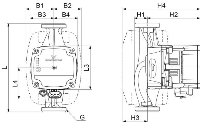
Рис. 24 Габаритные размеры ALPHA1 L XX-80
